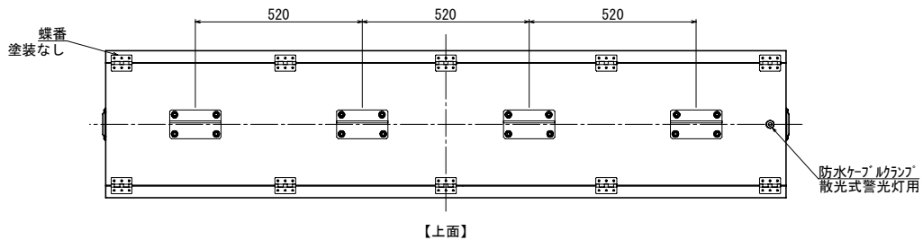
【上面】
