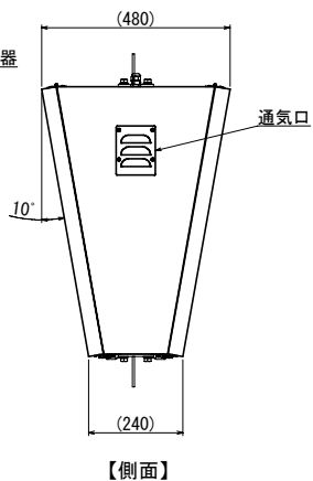
【側面】
