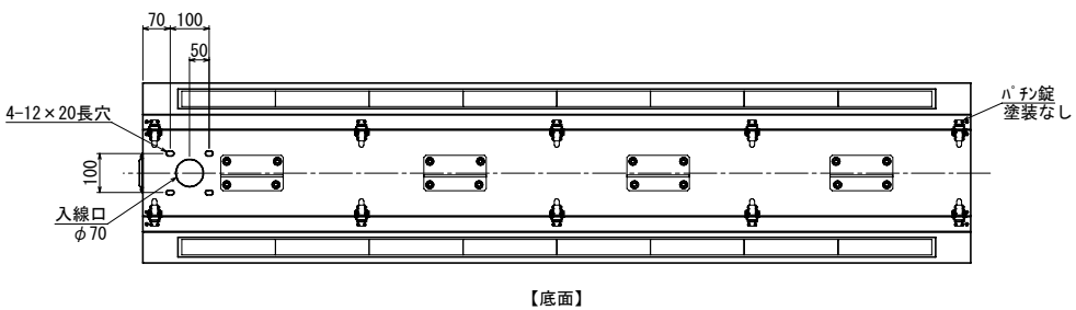
【底面】
