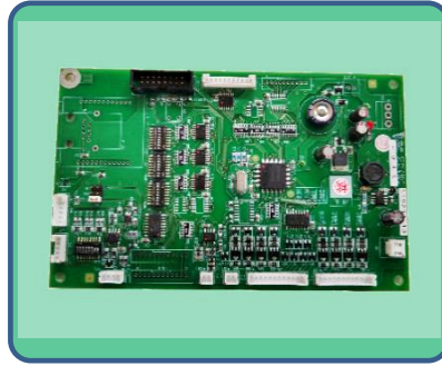
16ドットLED制御基板 シリアル通信モジュール搭載
