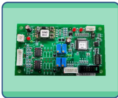
アナログ (電流、電圧) ⇒ シリアル変換基板
