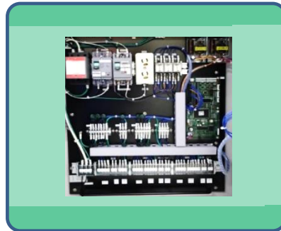
制御装置内実装写真
