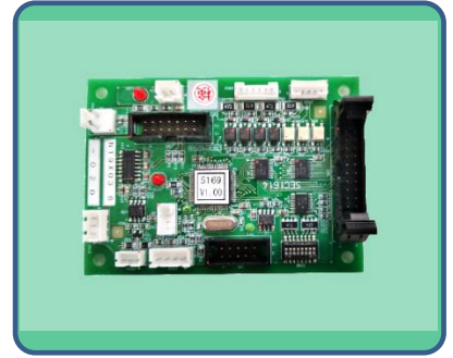
7セグメントLED制御基板 シリアル通信モジュール搭載
